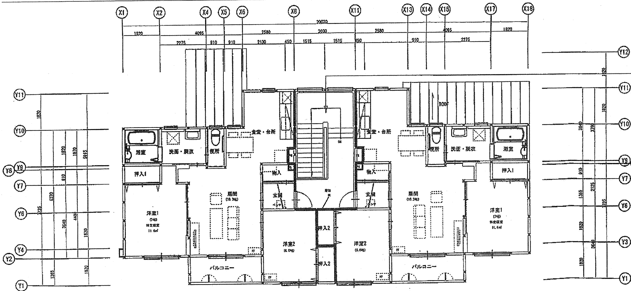
2階平面図
