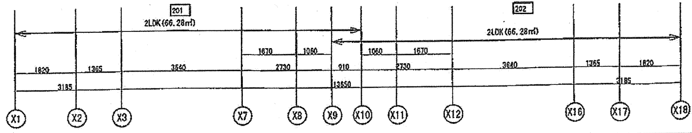
2階平面図
