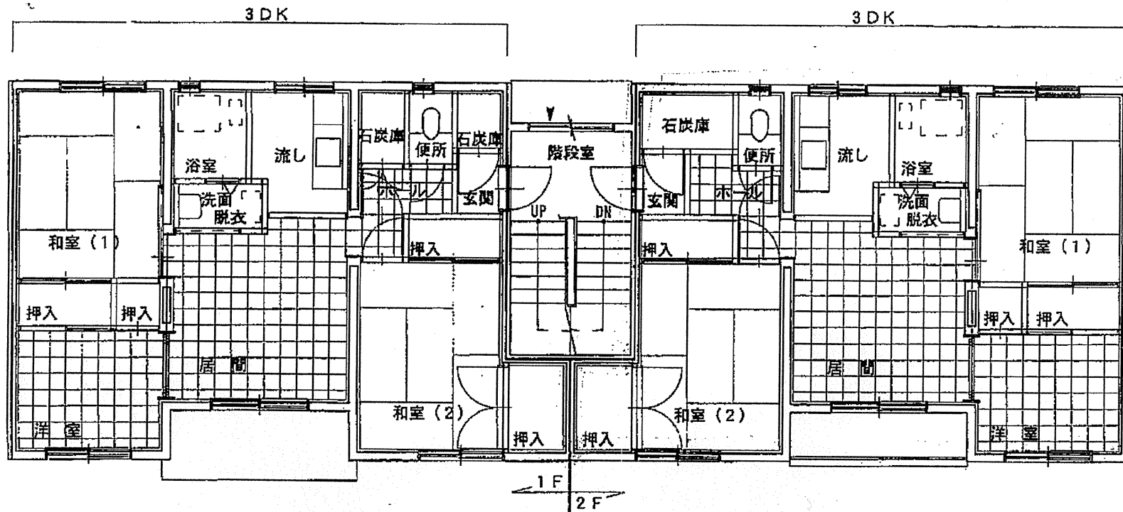
1 階 平 面 図
